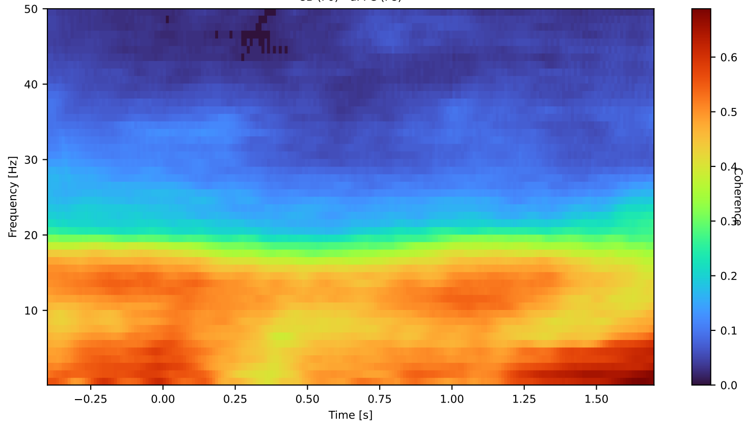
8B (F0) - dPFC (F8)
